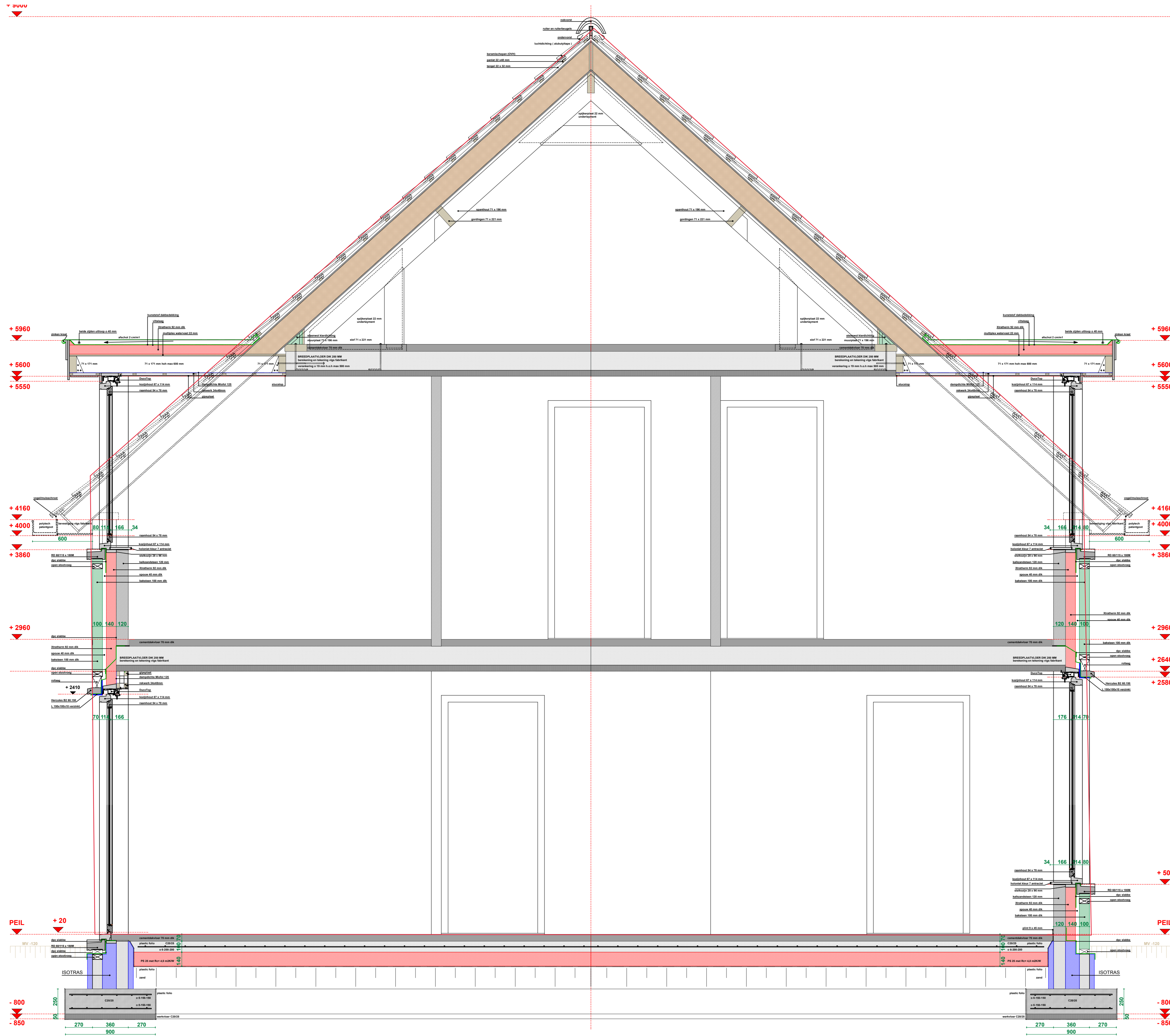
DOORSNEDE A-A
